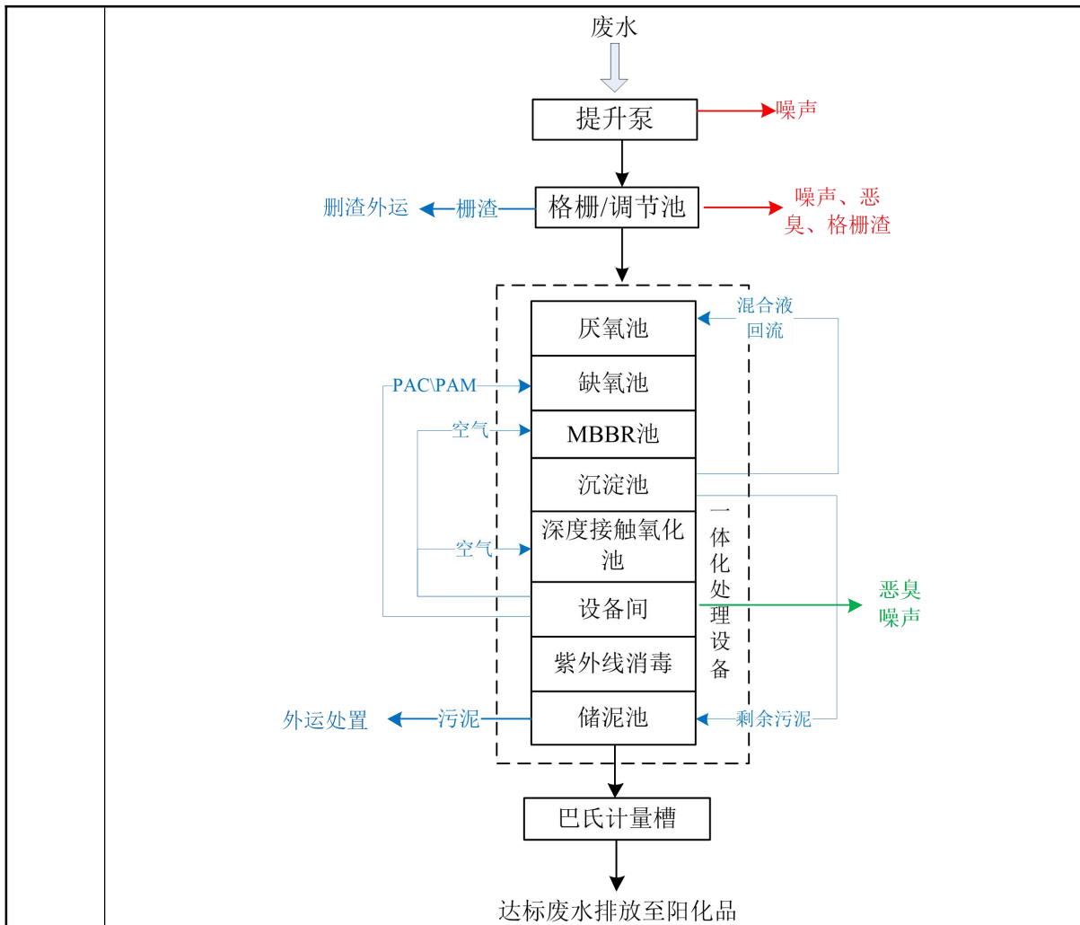
图 2-1 工艺流程图
